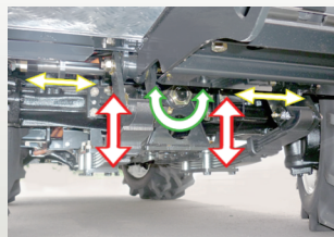
快適ハイブリッドサスペンション (黄色の⇄は、パワステ用油圧シリンダー)
