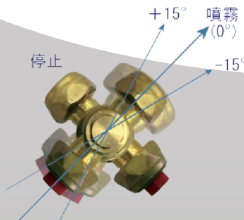
金属製スイッチノズル (上から 広角・標準・停止)
